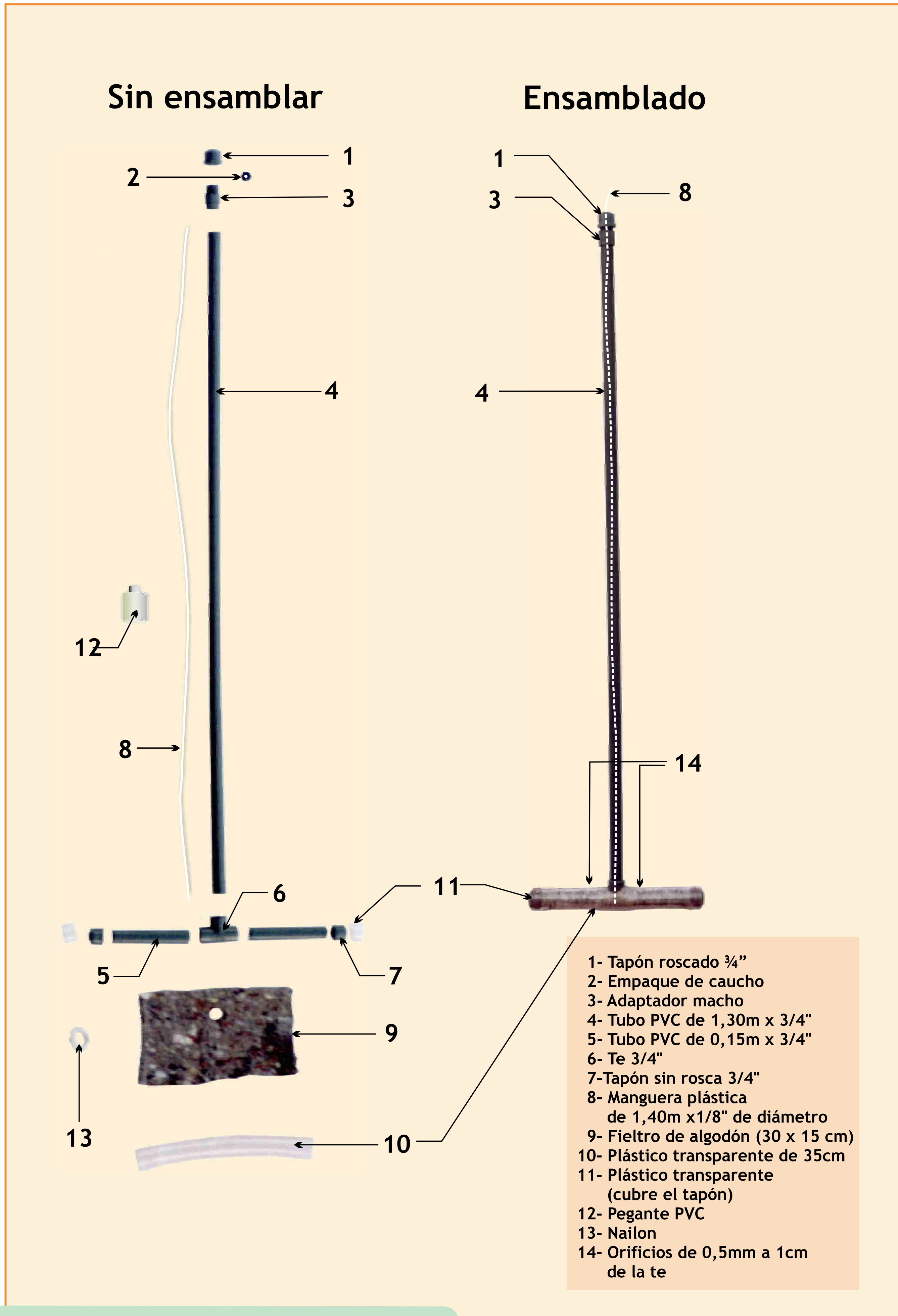
Figura 5.17. Componentes del selector de arvenses (Rivera, 2000).
