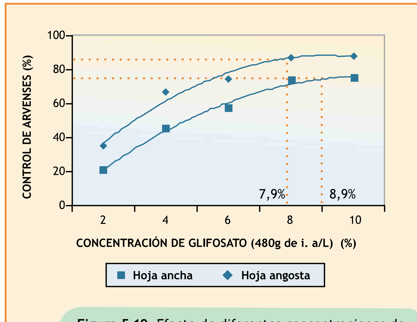
Figura 5.19. Efecto de diferentes concentraciones de glifosato aplicadas con el selector de arvenses sobre la eficacia del control (Salazar e Hincapié, 2003).
