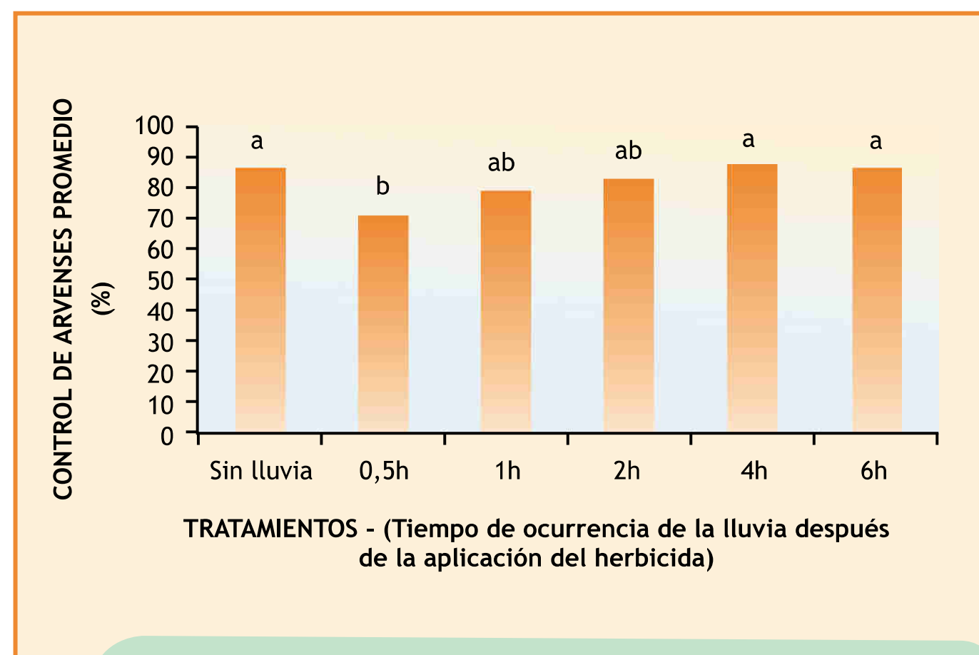
Figura 5.21. Efecto de una lluvia simulada de 60 mm/h sobre el control de arvenses con selector (Tratamientos acompañados con letras iguales no difieren estadísticamente) (Salazar e Hincapié, 2003).
