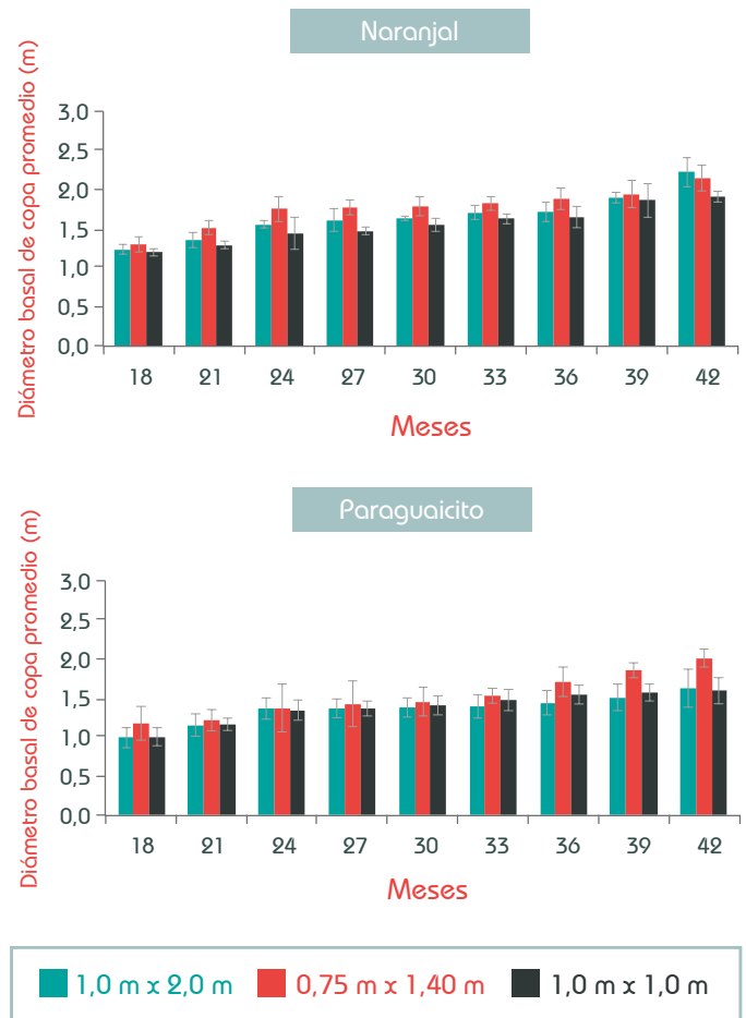
Figura 7. Promedio del diámetro basal de la copa de las plantas en las Estaciones Experimentales Naranjal y Paraguaicito. Las barras indican intervalos para la media con un coeficiente de confianza del 95%.
