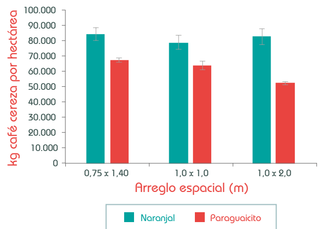
Figura 8. Producción de café cereza acumulada (kg.ha -1 ) en las Estaciones Experimentales Naranjal y Paraguaicito.
