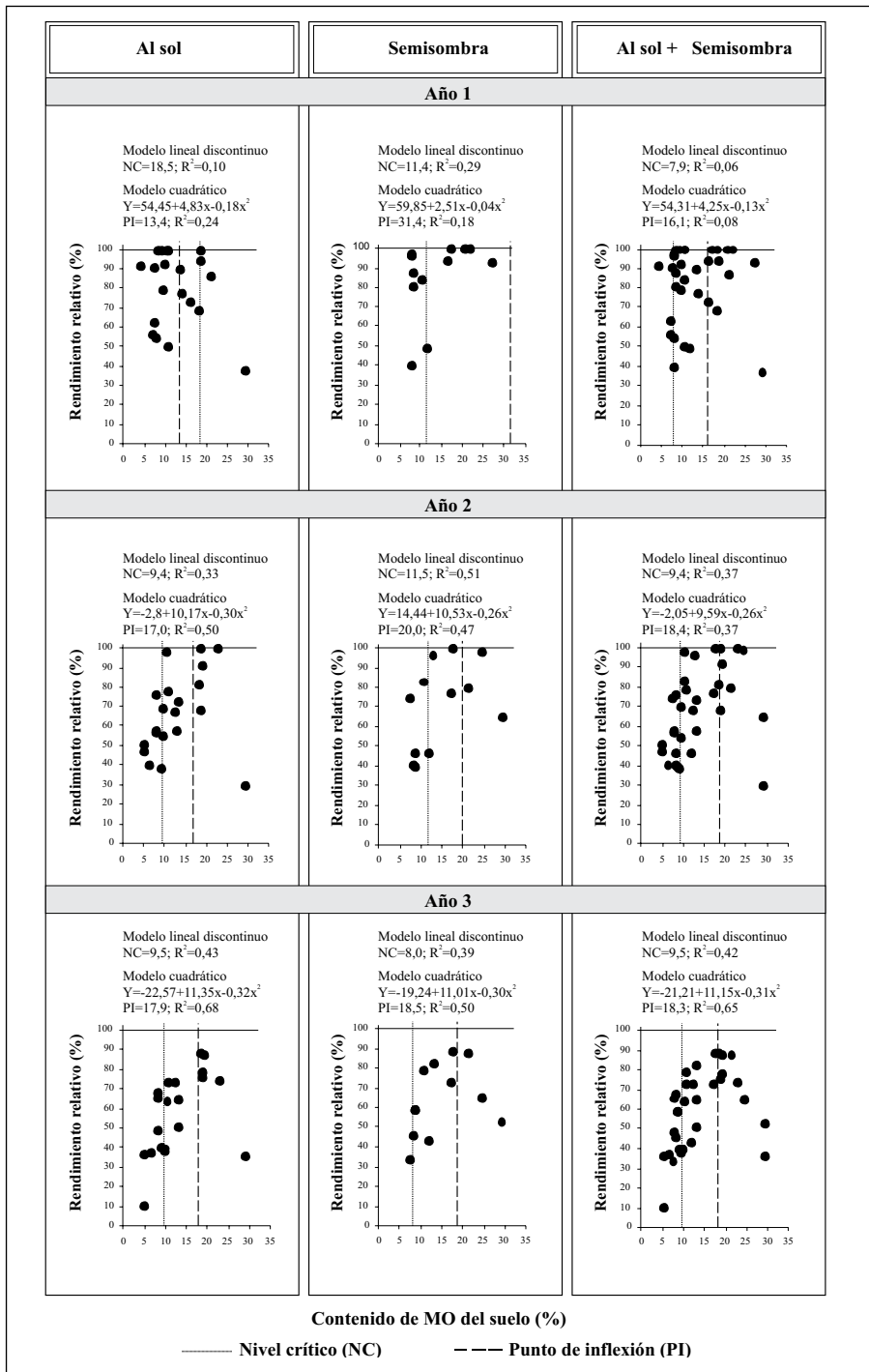
Figura 3. Relación entre el contenido de la MO del suelo y el rendimiento relativo de café al sol y bajo semisombra para tres años.
