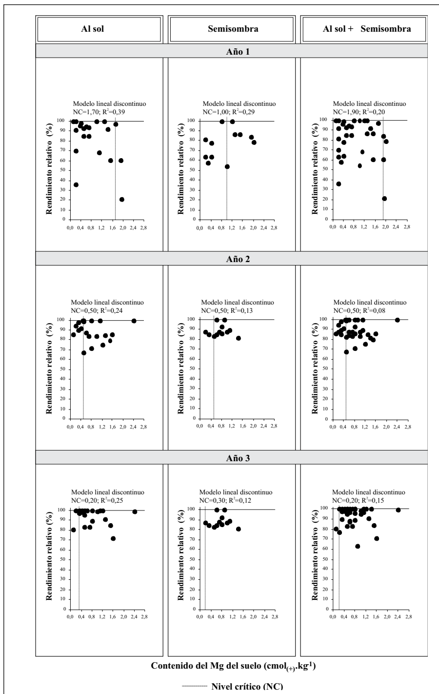
Figura 6. Relación entre el contenido del Mg del suelo y el rendimiento relativo de café al sol y bajo semisombra para tres años.
