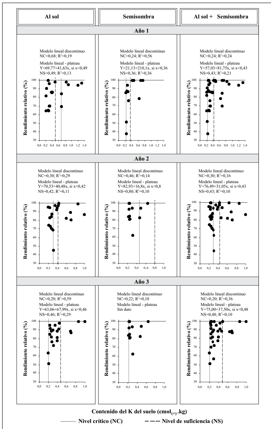
Figura 5. Relación entre el contenido del K del suelo y el rendimiento relativo de café al sol y bajo semisombra para tres años.
