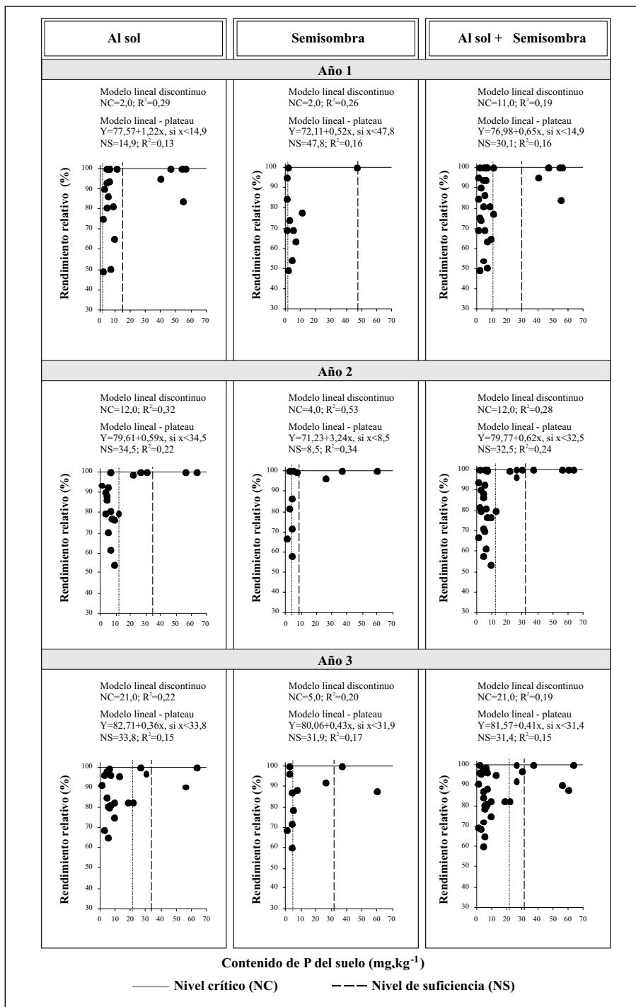
Figura 4. Relación entre el contenido de P del suelo y el rendimiento relativo de café al sol y bajo semisombra para tres años.
