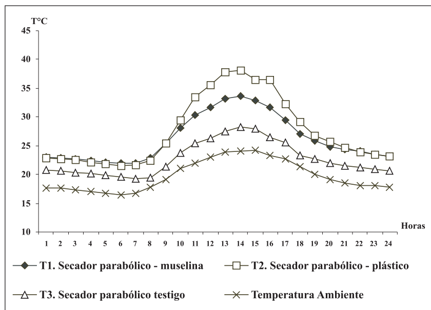
Figura 2. Promedio de temperatura horaria (24 horas) en los distintos secadores parabólicos durante los seis días del secado del café pergamino.
