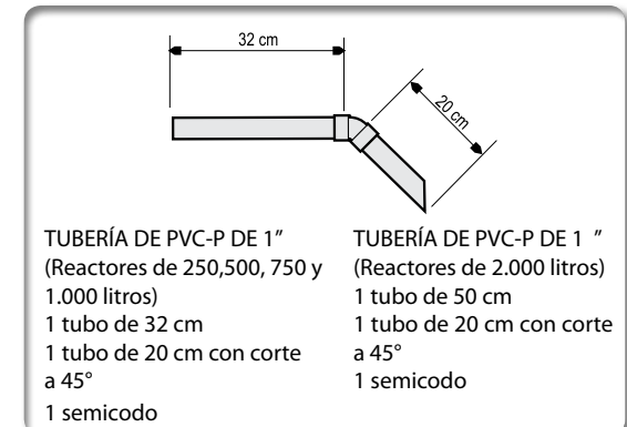
Figura 35. Dispositivo de salida del reactor metanogénico.
